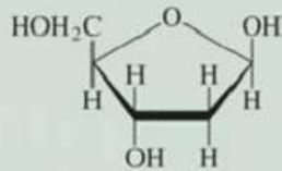
Deoxyribose
