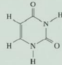
Uracil
