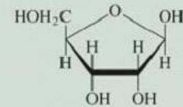
Ribose
